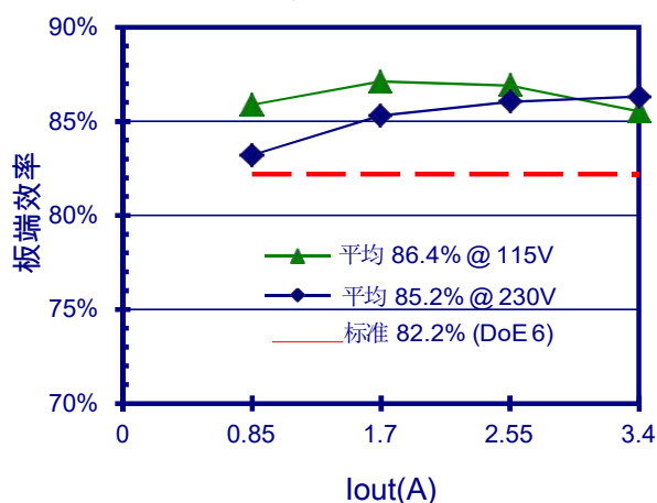
5V-3.4A (FT8393MDD1+FT8370CP)
