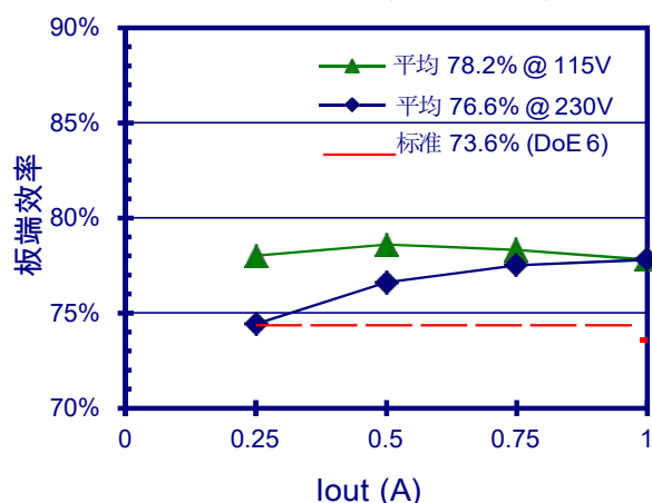
5V-1A (FT839NB1)
