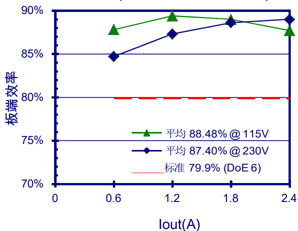
5V-2.4A (FT8393MB1+FT8370B)
