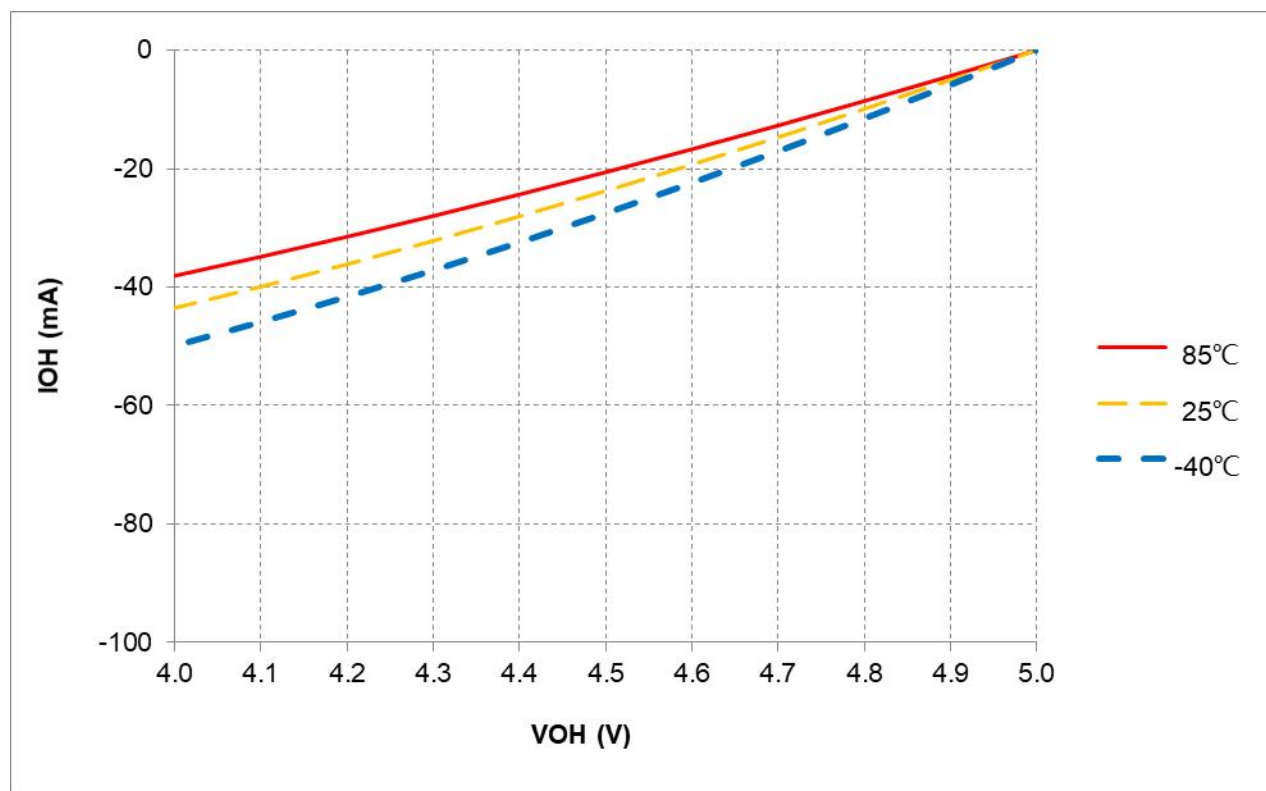
图 17-7 I_{OH} vs. V_{OH} @L2 = -18\text{mA} , V_{DD} = 5\text{V}
