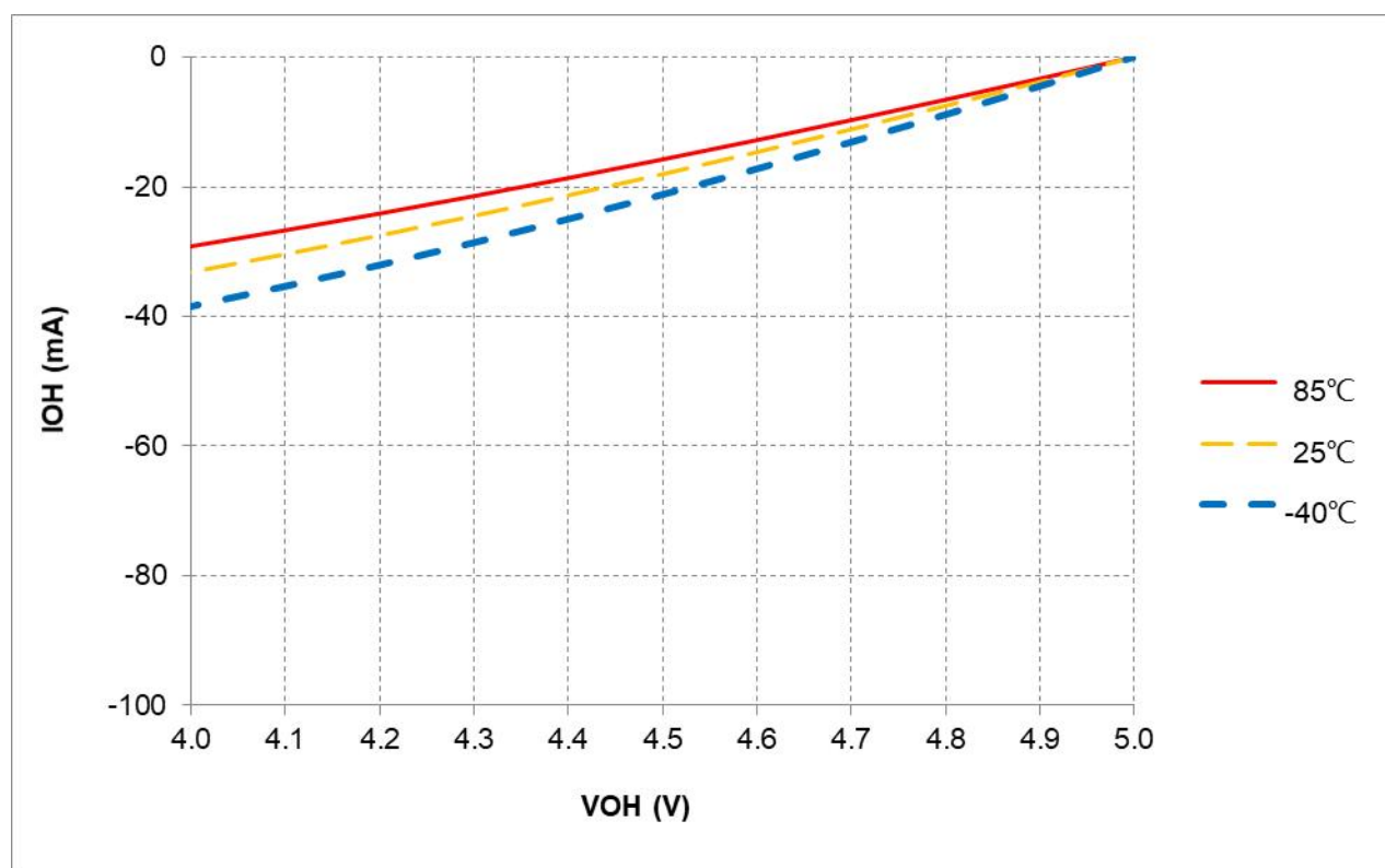
图 17-8 I_{OH} vs. V_{OH} @L3 = -24\text{mA} , V_{DD} = 5\text{V}
