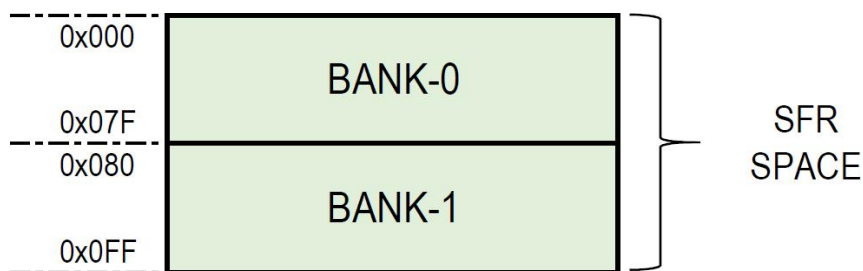
图 15-2 间接寻址
