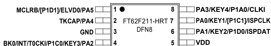
图 1-5 DFN8 3
