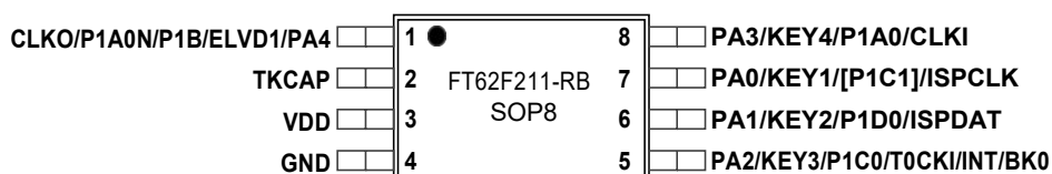
图 1-4 SOP8
