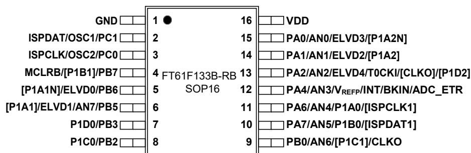
图 1-7 SOP16 2
