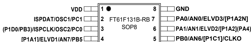
图 1-2 SOP8 1 2
