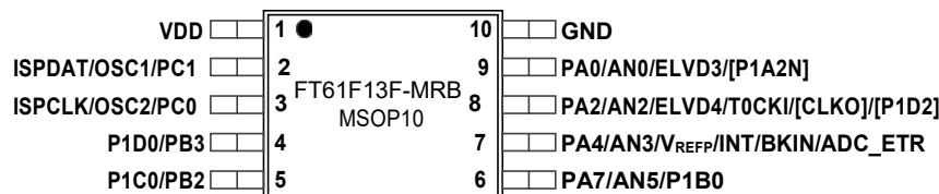
图 1-4 MSOP10 2
