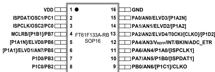
图 1-6 SOP16 2
