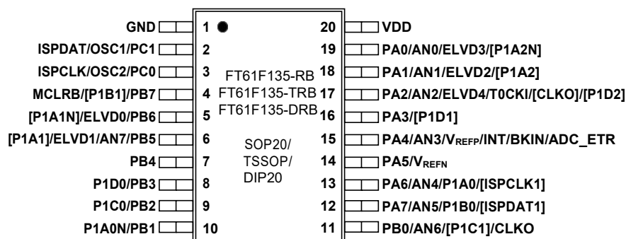
图 1-8 SOP20 / TSSOP20 / DIP20
