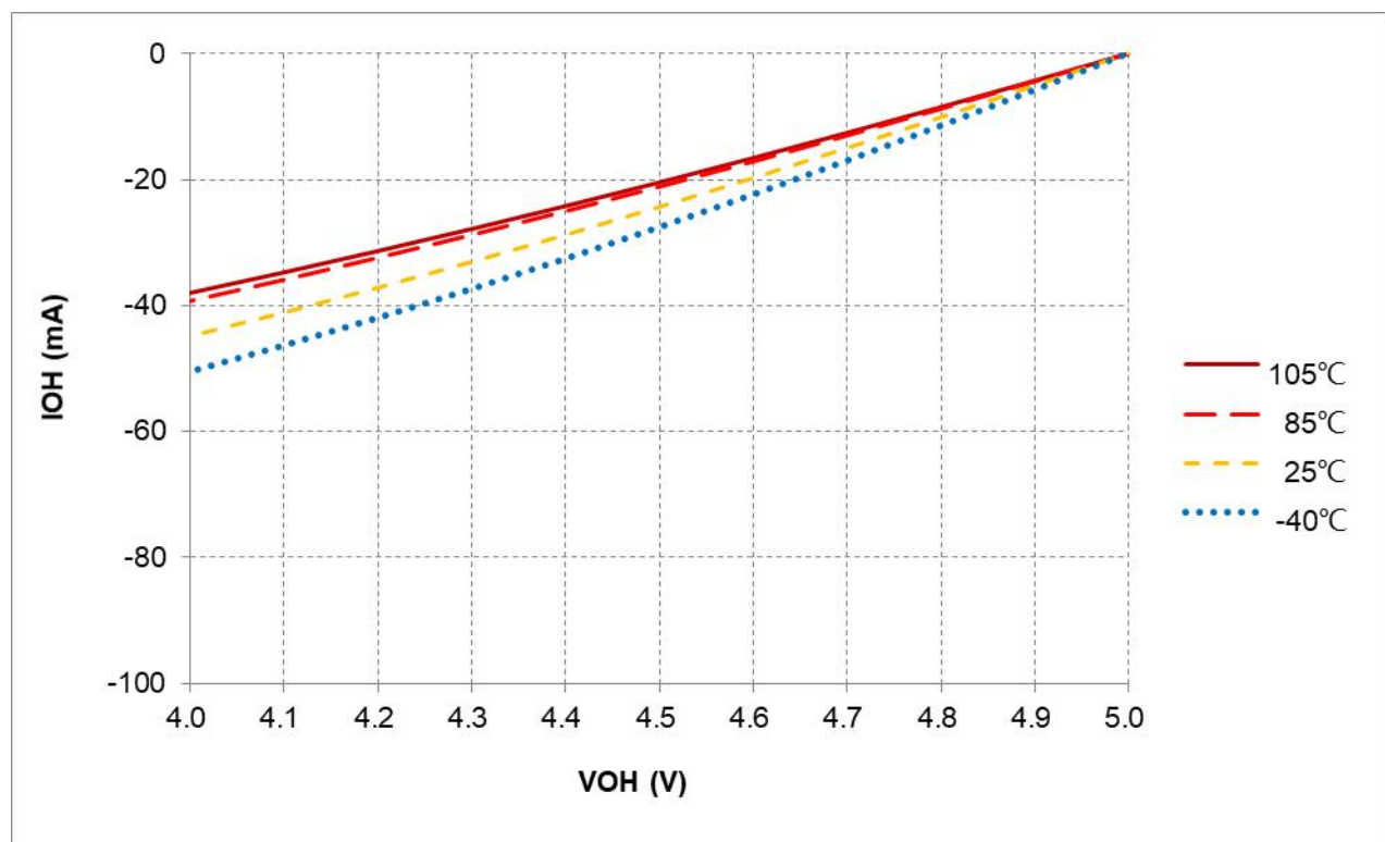
图 3-8 I_{OH} vs. V_{OH} @L3 = -24\text{mA} , V_{DD} = 5\text{V}
