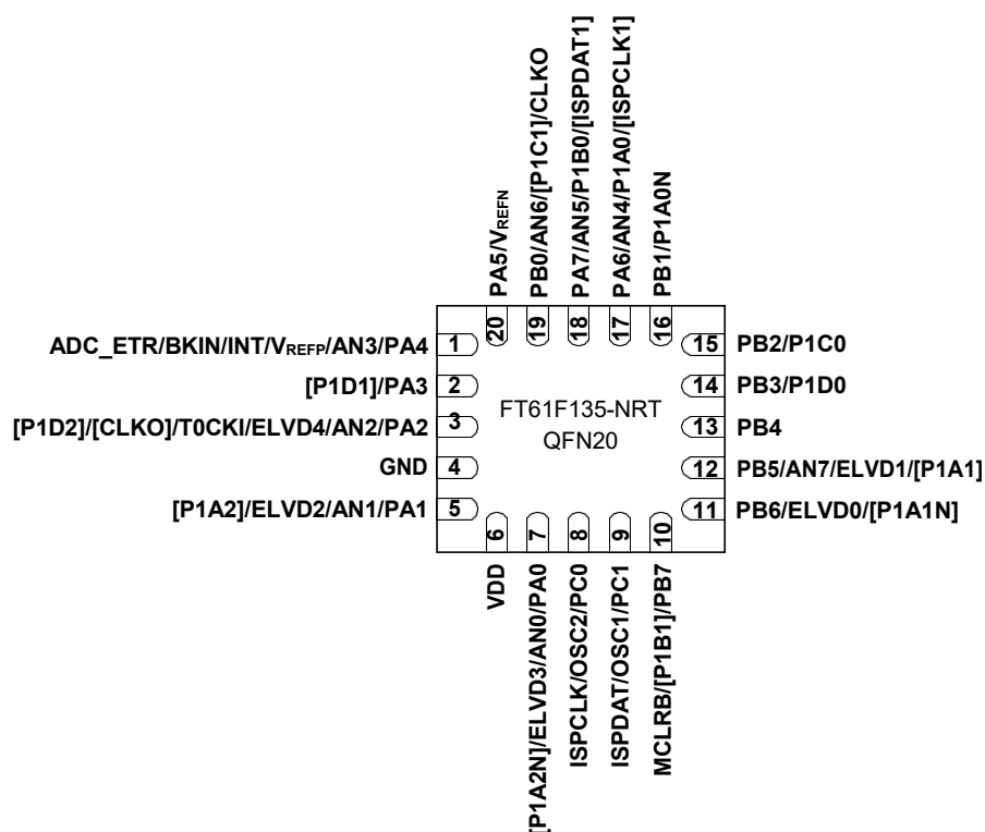
图 1-9 QFN20 4
