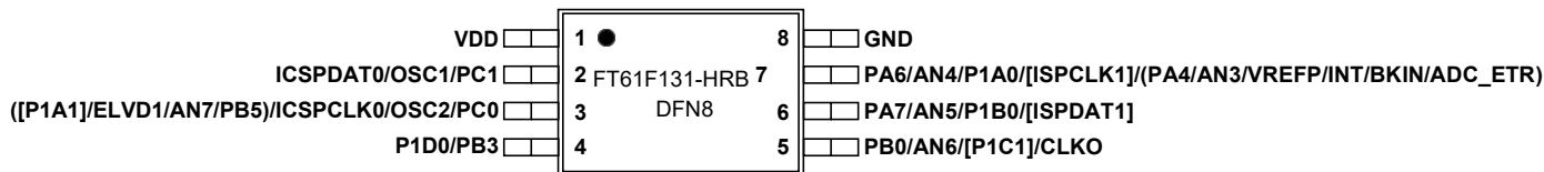
图 1-3 DFN8 2 3
