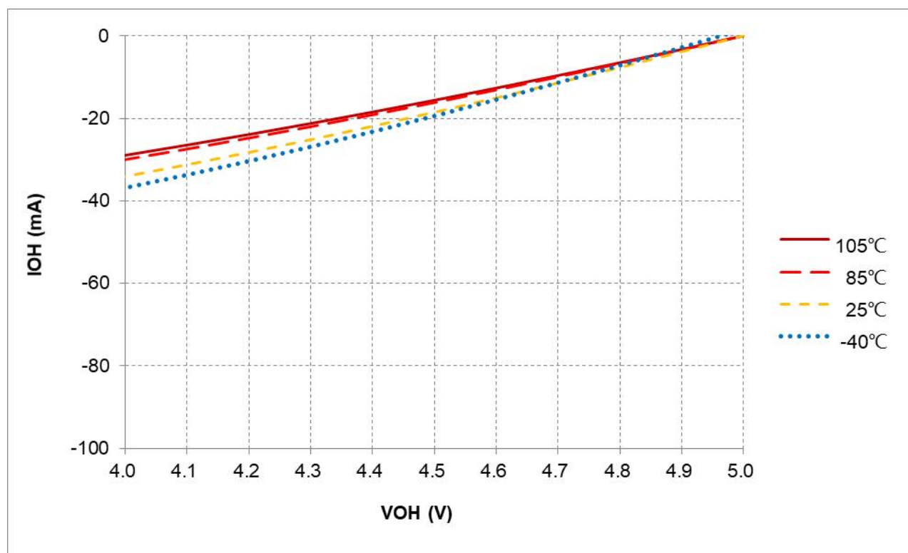
图 3-7 I_{OH} vs. V_{OH} @L2 = -18\text{mA} , V_{DD} = 5\text{V}
