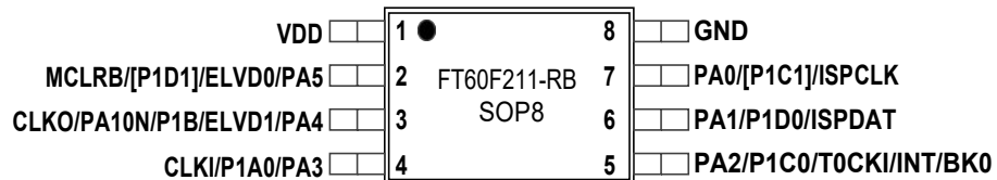
图 1-3 SOP8
