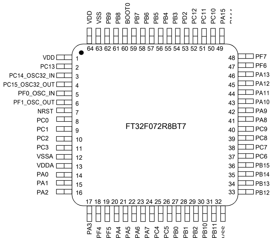
图 4-2 LQF64-B 引脚分配
