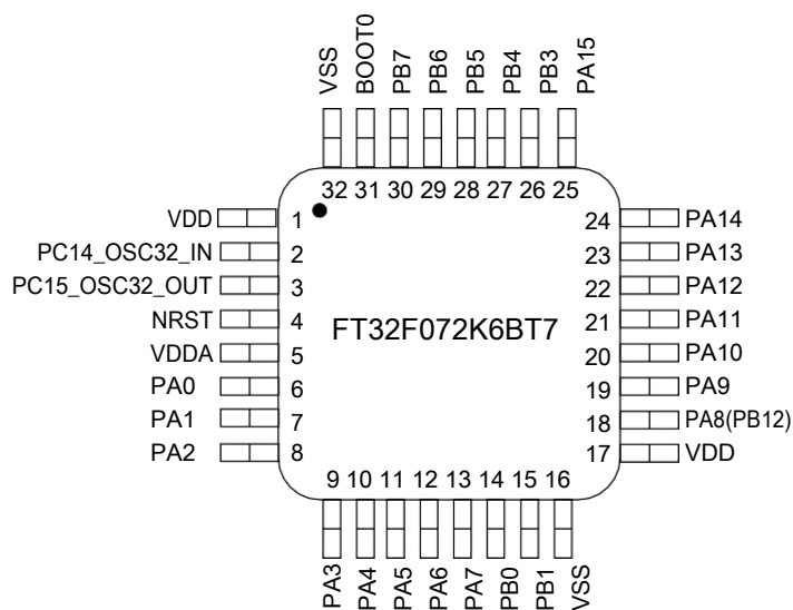
图 4-4 LQFP32 引脚分配 3
