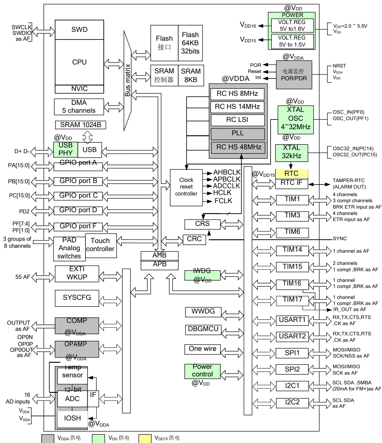
图 2-1 系统框图
