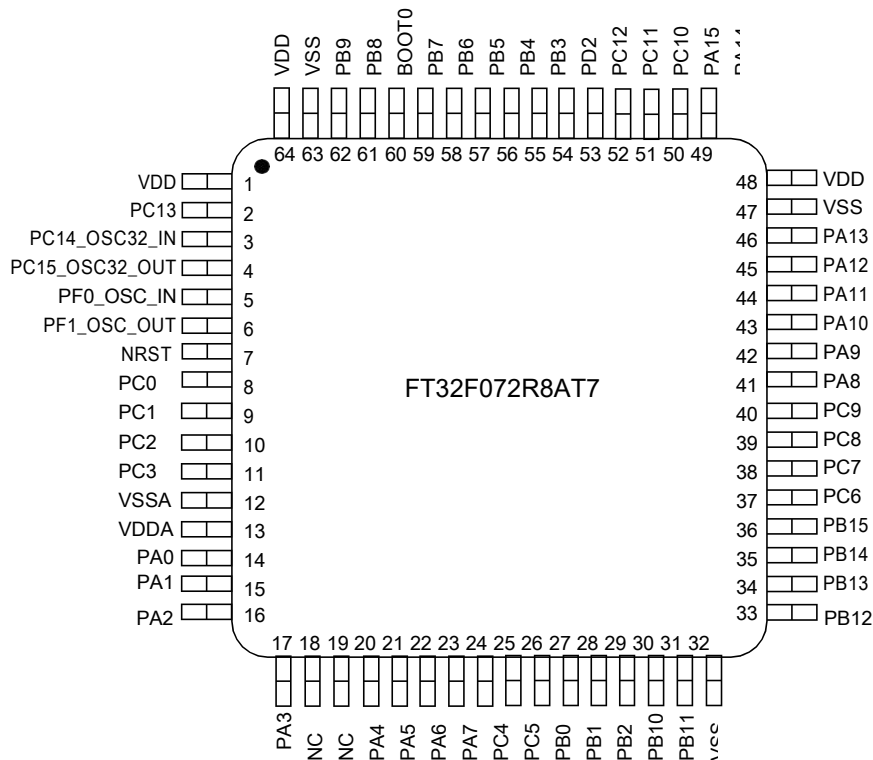
图 4-1 LQF64-A 引脚分配
