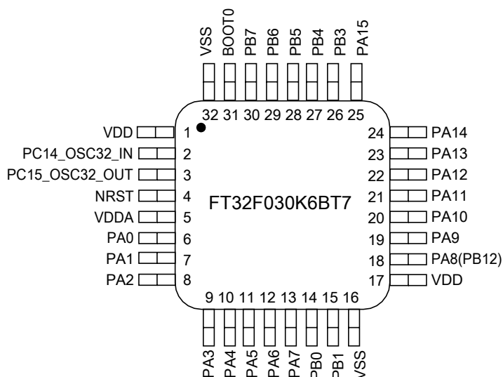
图 4-4 LQFP32 (A) 引脚分配 4
