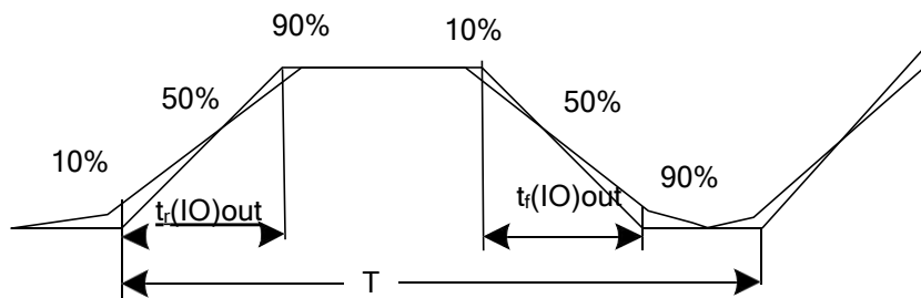
图 6-9 I/O交流特性定义
