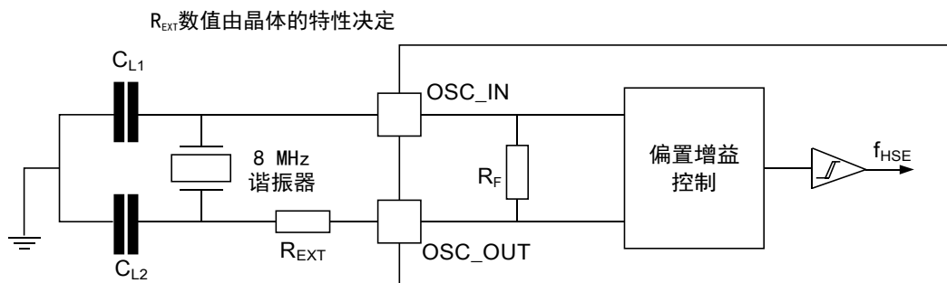
图 6-7 使用 8MHz 晶体的典型应用
