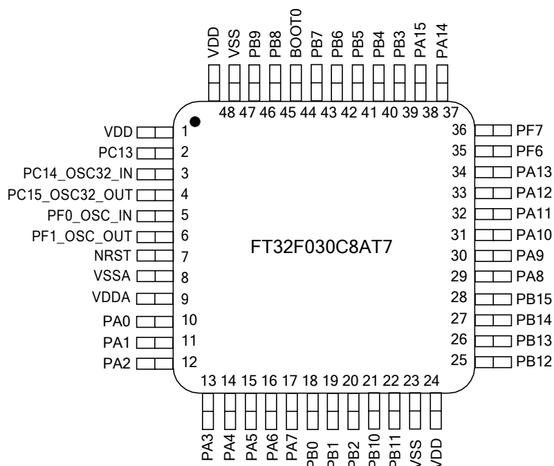
图 4-2 LQFP48 引脚分配
