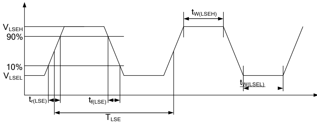
图 6-6 外部低速时钟源交流时序图使
