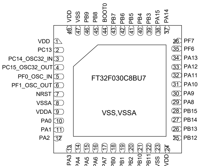
图 4-7 QFN48 引脚分配
