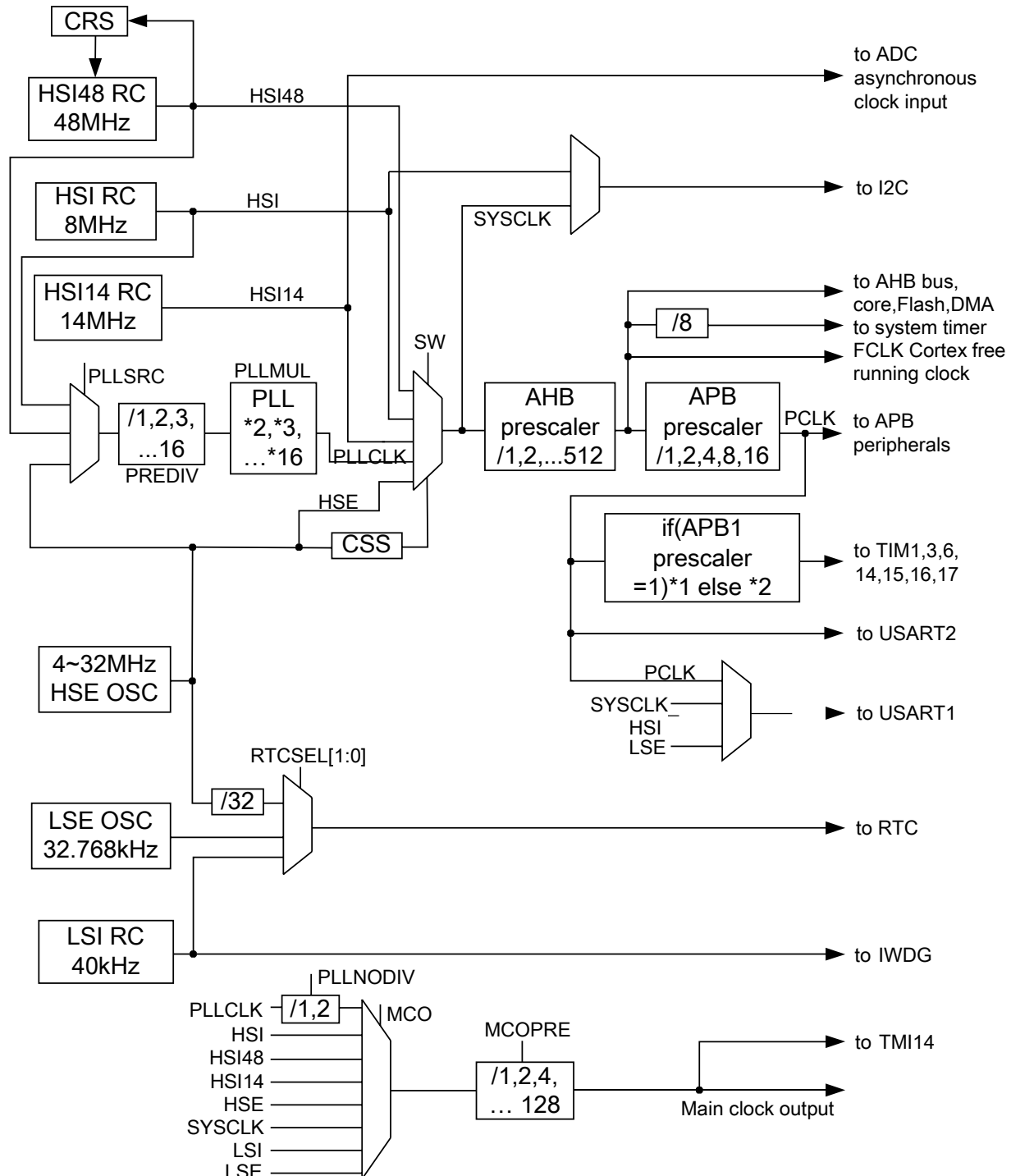
图 3-1 时钟框图
