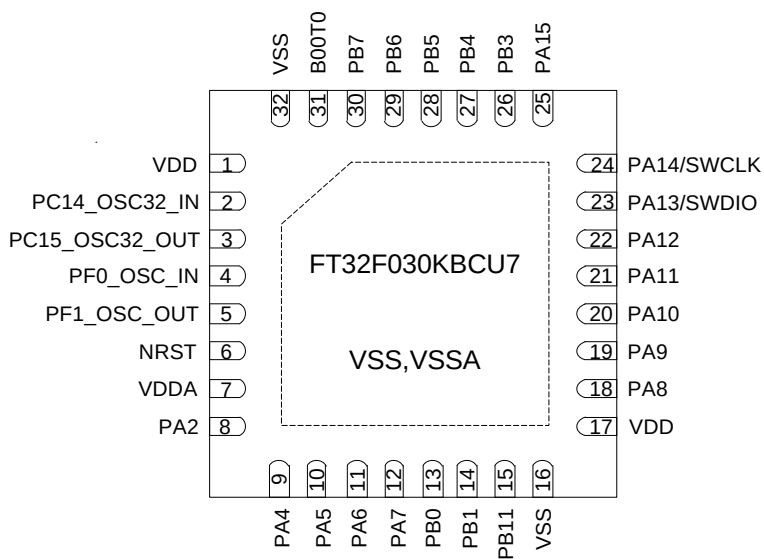
图 4.2 QFN32 引脚分配
