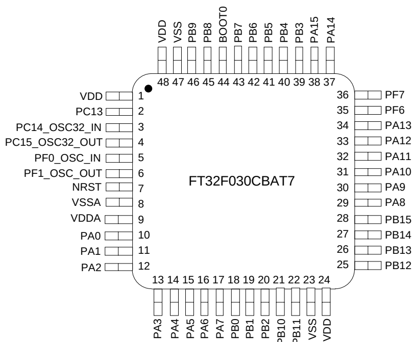
图 4.1 LQF48 引脚分配
