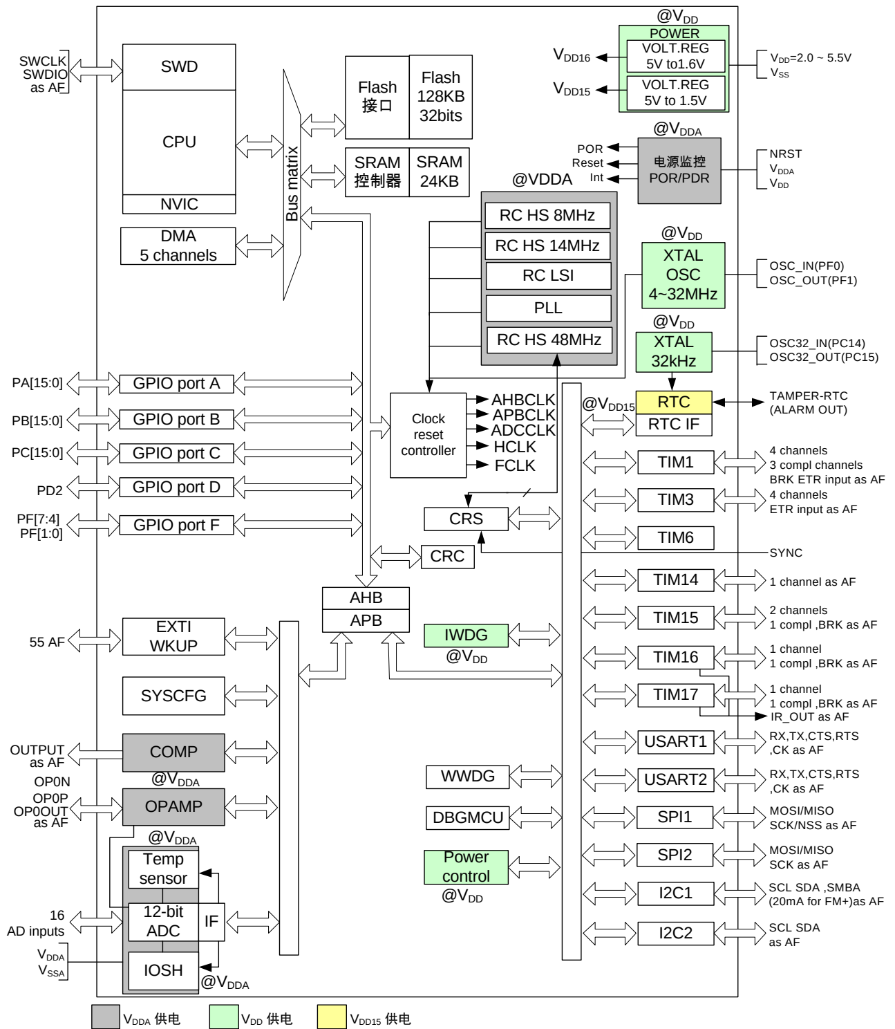
图 2.1 系统框图
