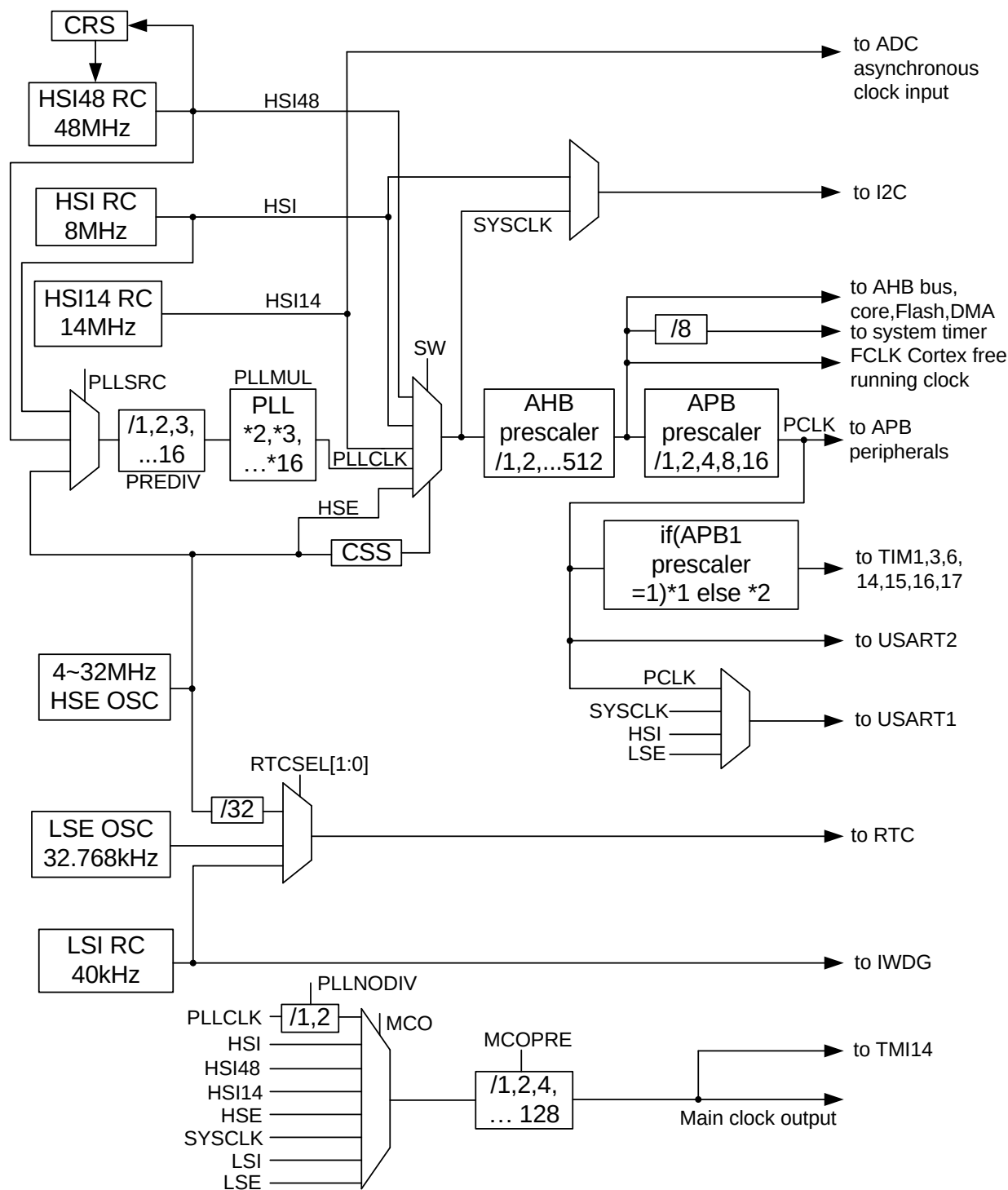
图 3.1 时钟框图
